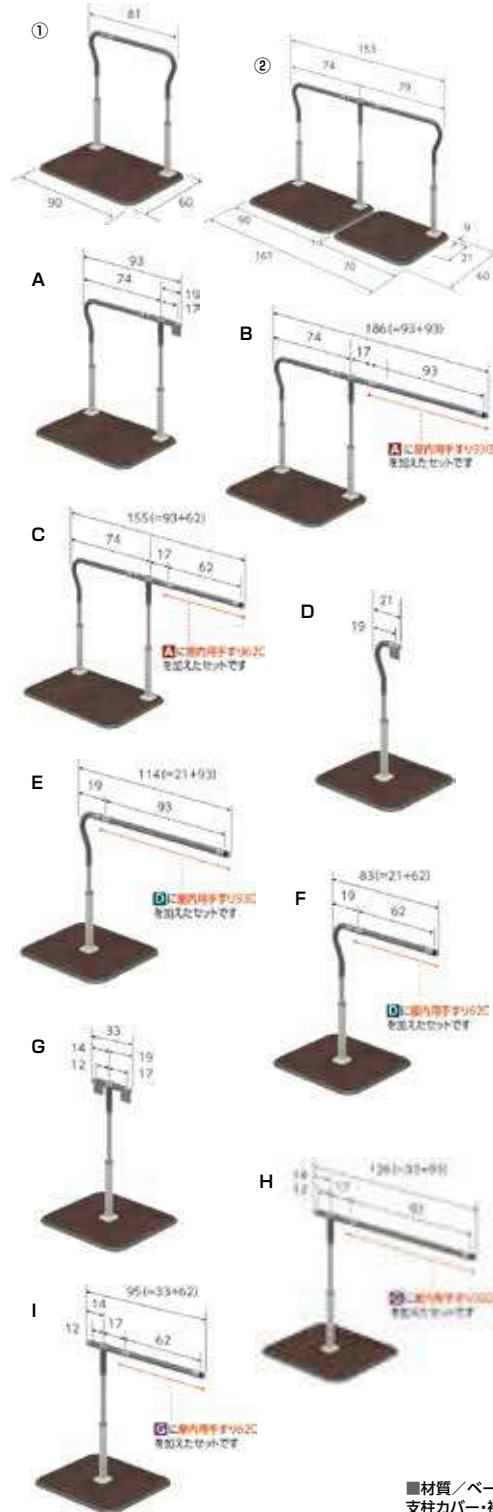
A + F 手すり長さ173cm 手すり高さ 70~85cm(2.5cmピッチ7段階)
